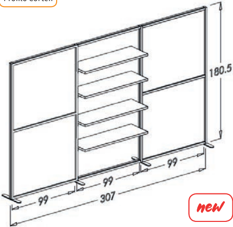
Profilo Corten
